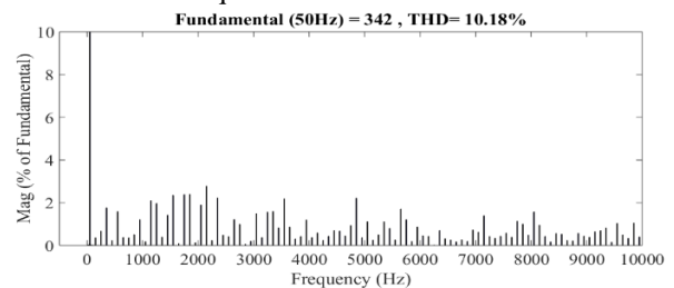
a) PDSPWM
