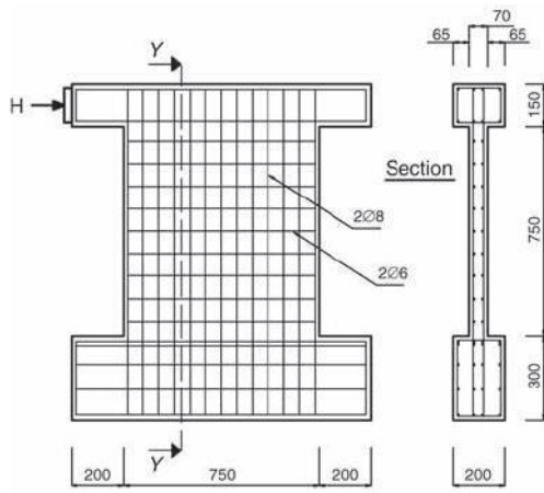
Figure 7. Lefas and Kotsivos wall SW11.
